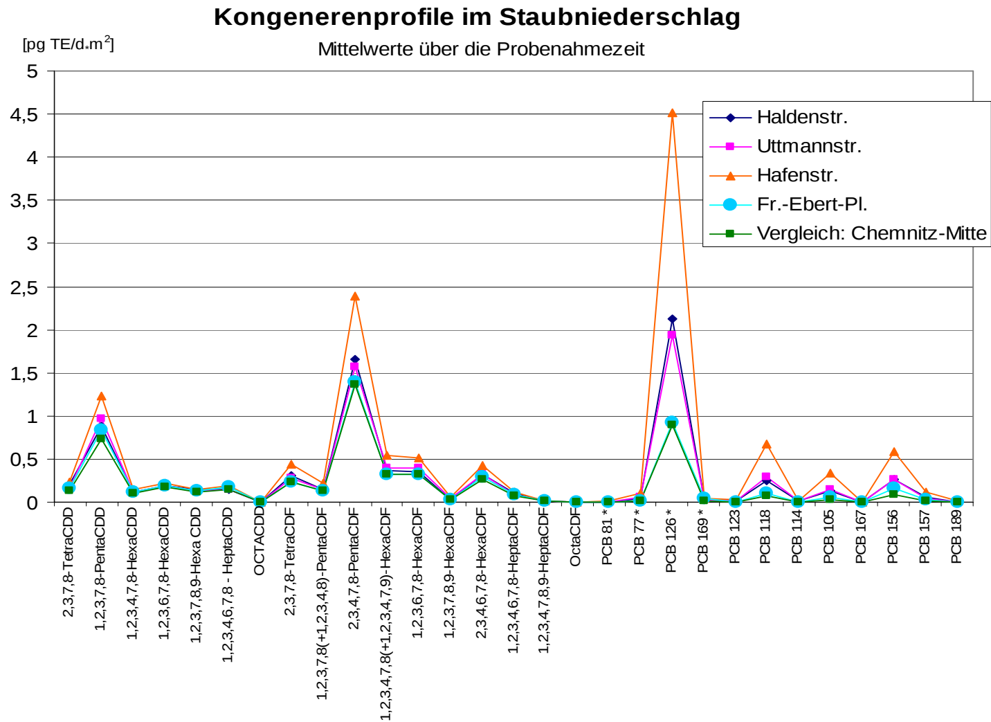
Abb. 8: Kongenerenprofile im Staubniederschlag (Mittelwerte; Halden-, Uttmann- und Hafenstr. von September 2008 bis August 2009; Fr.-Ebert-Platz und Chemnitz-Mitte von Februar bis August 2009)
